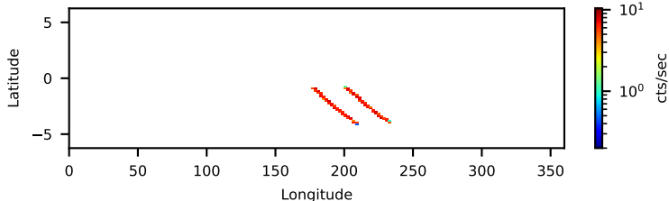
10502001010: 3 to 10 keV
