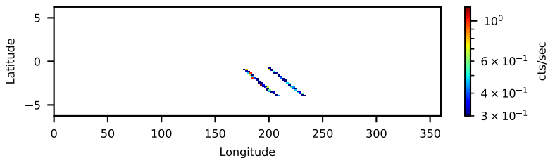
10502001010: 30 to 120 keV
