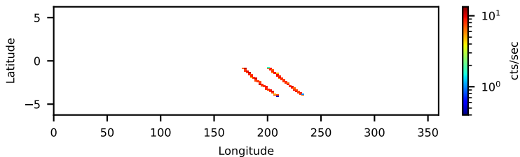
10502001010: 3 to 120 keV
