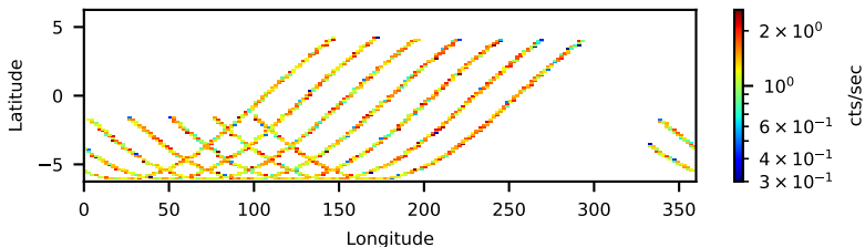
10402002004: 30 to 120 keV
