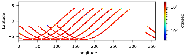
10402002004: 3 to 120 keV
