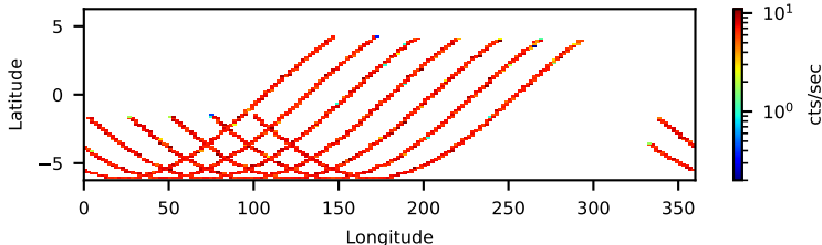
10402002004: 3 to 10 keV
