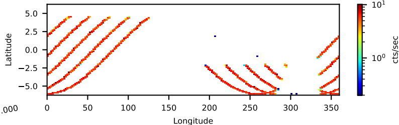
10402001006: 30 to 120 keV
