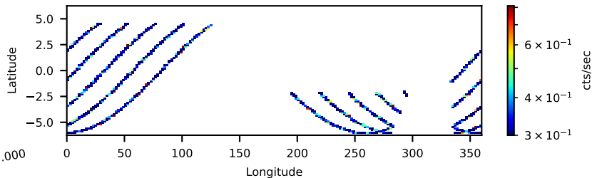
10402001006: 30 to 120 keV
