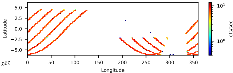
10402001006: 3 to 10 keV
