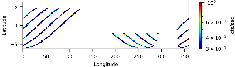
10402001006: 30 to 120 keV
