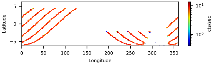
10402001006: 3 to 120 keV
