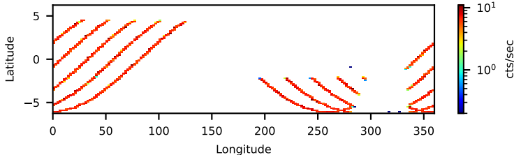
10402001006: 3 to 10 keV
