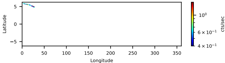
10310003001: 3 to 120 keV
