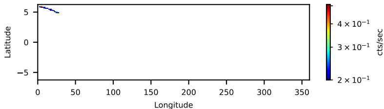
10310003001: 3 to 10 keV
