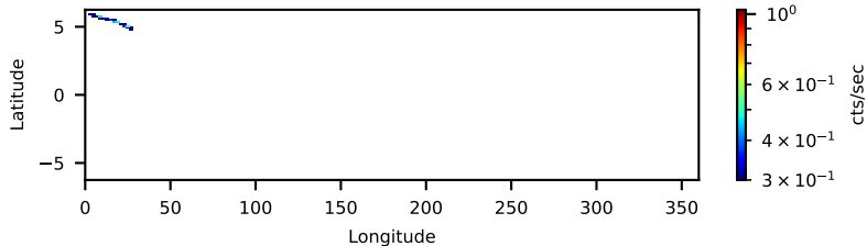
10310003001: 30 to 120 keV
