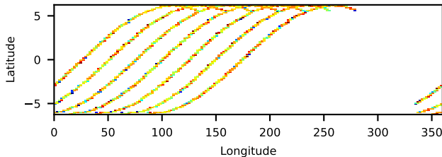
10210001002: 30 to 120 keV
