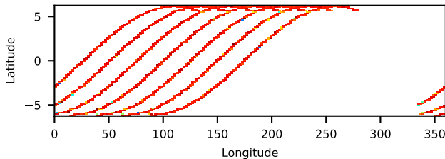
10210001002: 3 to 120 keV
