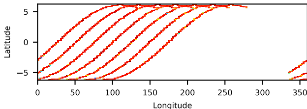
10210001002: 3 to 10 keV
