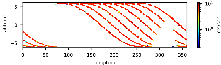
10110004002: 3 to 10 keV
