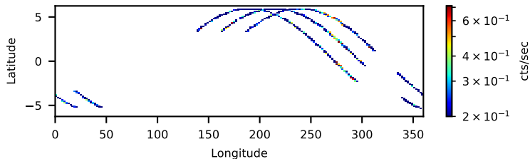
10060003001: 3 to 10 keV
