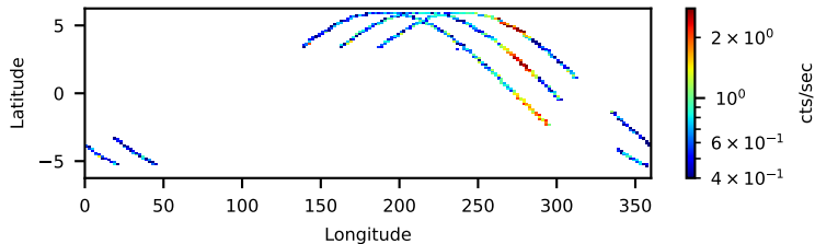
10060003001: 3 to 120 keV
