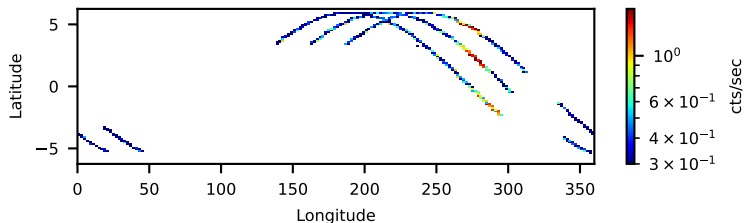
10060003001: 30 to 120 keV
