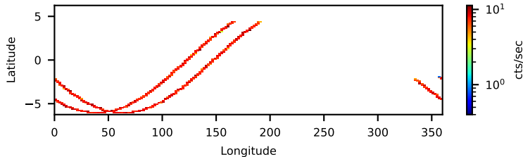
10013037008: 3 to 120 keV
