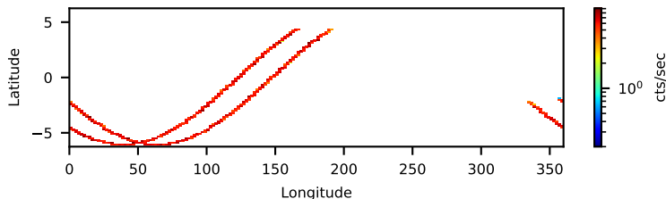
10013037008: 3 to 10 keV
