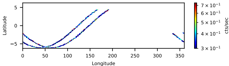
10013037008: 30 to 120 keV
