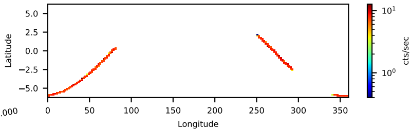
10013027002: 3 to 10 keV
