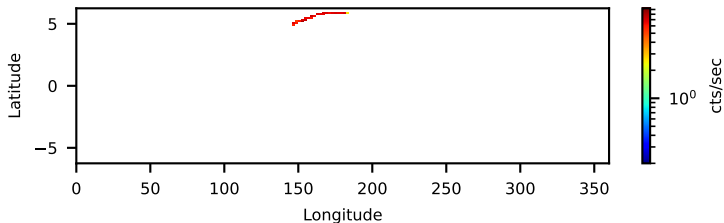
10013010001: 3 to 10 keV
