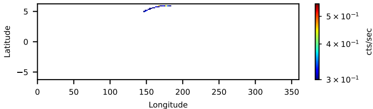
10013010001: 30 to 120 keV
