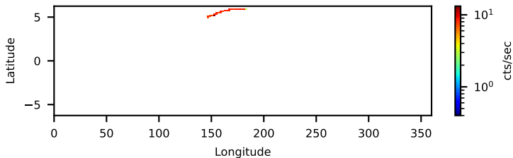
10013010001: 3 to 120 keV
