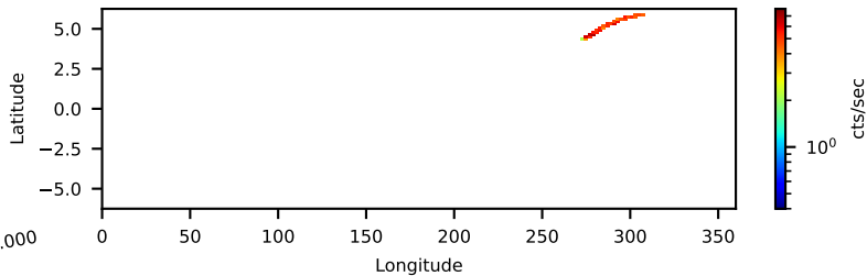
10013003001: 3 to 10 keV
