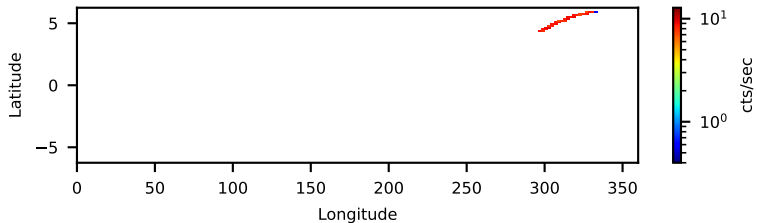
10013001001: 3 to 120 keV
