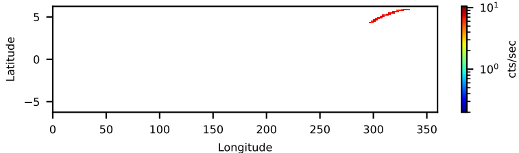
10013001001: 3 to 10 keV
