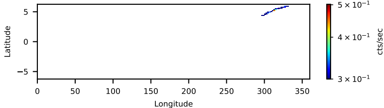
10013001001: 30 to 120 keV
