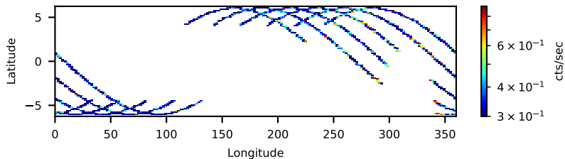
10002013003: 30 to 120 keV
