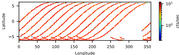
10002001006: 3 to 10 keV
