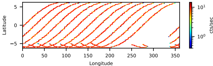
10002001006: 3 to 120 keV
