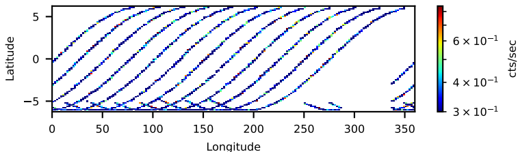
10002001006: 30 to 120 keV
