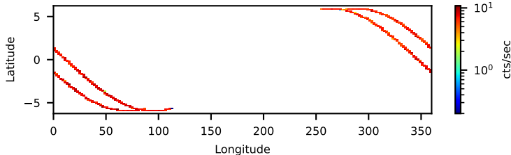
10002001002: 3 to 10 keV
